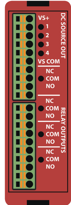
EZLGX-IO-4DCOP4RLO
