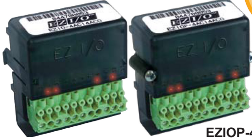
EZIO-4DCI4DCOP Snap-in
